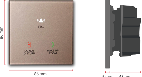
1 Conjoined
